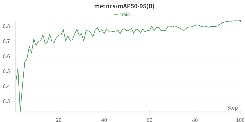
Figure 2. YOLO11 mAP50-95.
