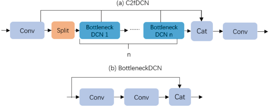
Fig. 4. C2fDCN module
